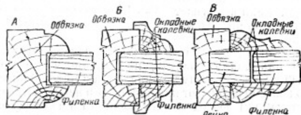
Рис. 109. Соединение филенки с обвязками
