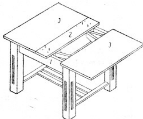
Рис. 115. Раздвижной обеденный стол: 1—подсто́лье; 2—мостик; 3—выдвижные полукрышки (верхняя доска снята)
