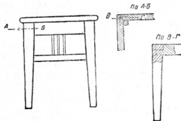
Рис. 112. Табурет
