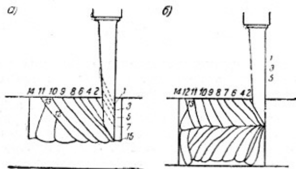
Рис. 46. Долбление гнезд:
