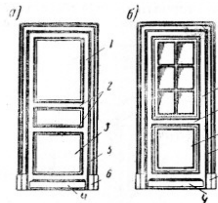
Рис. 108. Филечатые двери:
