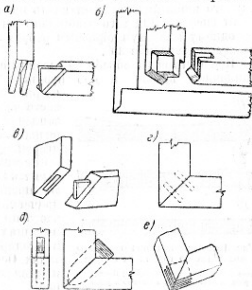
Рис. 99. Угловые соединения на ус:
