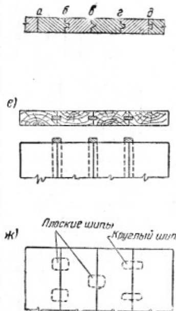
Рис. 101. Сплачивание щитов:
