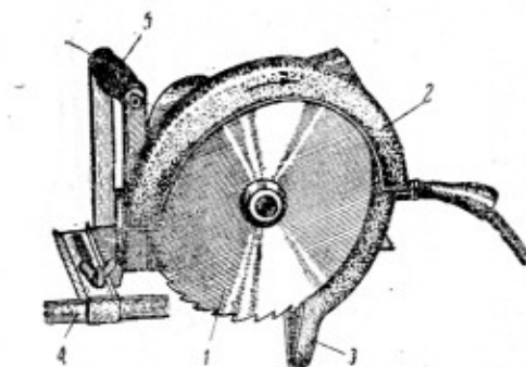
Рис. 90. Дискосвая безредукторная электропила ДПА-27:
