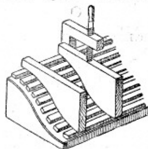
Рис. 138. Фанерование изогнутой поверхности при помощи реечной цулаги
