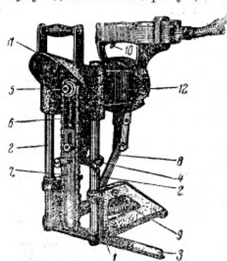
Рис. 94. Электродолбежник ДА-27:
