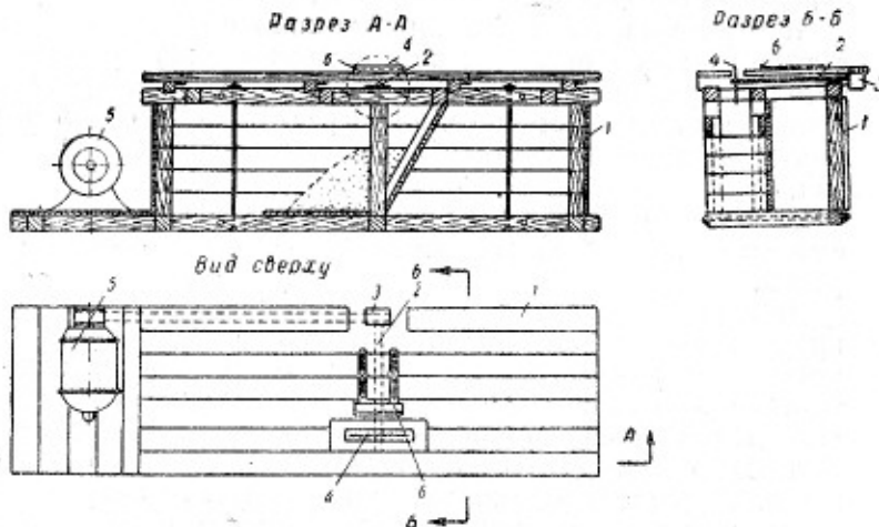
Рис. 60. Циркулярная пила:
