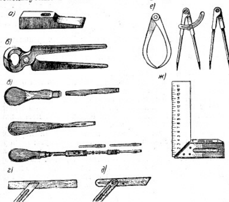
Рис. 55. Вспомогательные и контрольно-измерительные инструменты:
