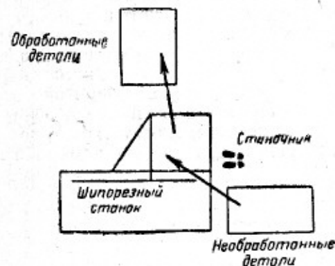
Рис. 146. Схема организации рабочего места у шипорезного станка
