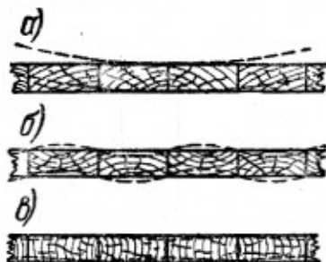
Рис. 100. Способы подбора делянок шипа по годичным слоям:
