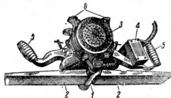
Рис. 91. Электрорубанок ЭРБ-100:
