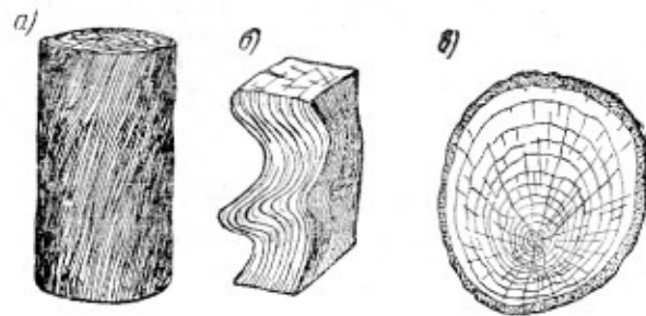
Рис. 12. Неправильности строения древесины: а — косошлой; б — сплюснутости; в — knots
