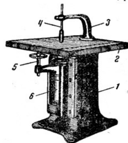
Рис. 70. Фрезерный станок:
