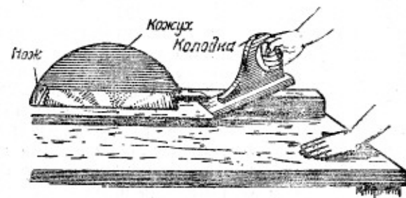
Рис. 61. Расклинивающий нож, защитный кожух и предохранительная колодка
