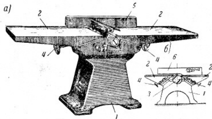
Рис. 67. Фуговочный станок:
