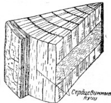
Рис. 3. Серцевинные лучи
