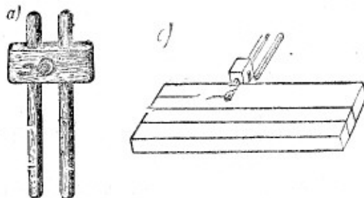
Рис. 36. Рейсмус а и разметка рейсмусом б
