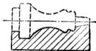
Рис. 85. Шаблон для проверки точного профиля
