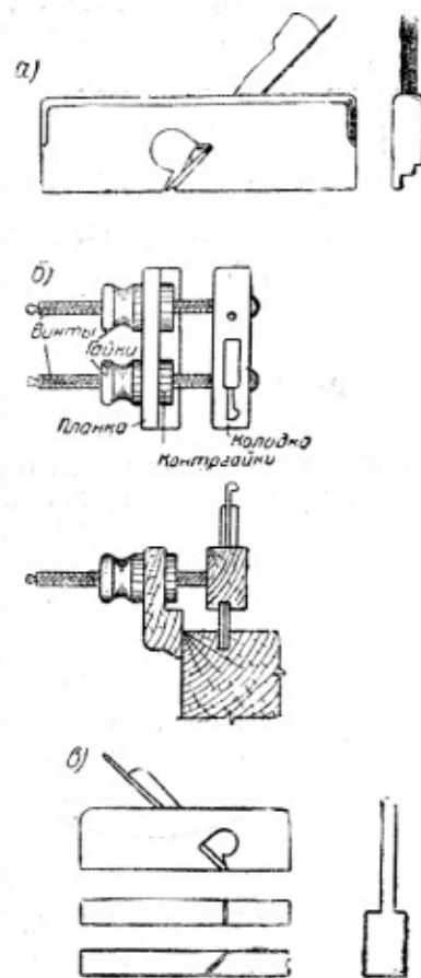
Рис. 39. Фигурные рубанки:
