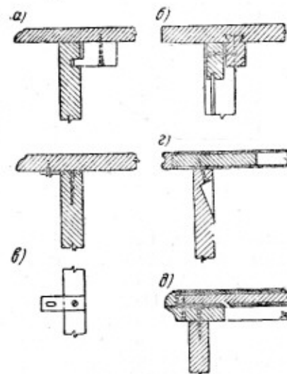
Рис. 118. Способы крепления крышки стола к подстолью:
