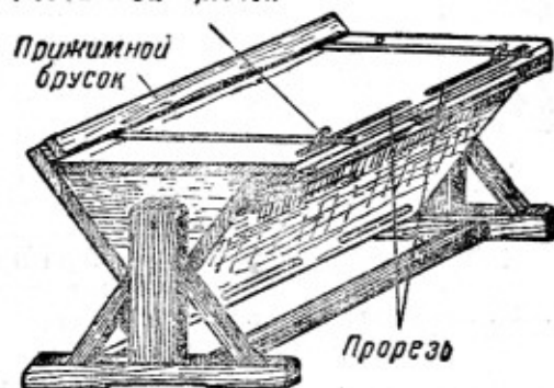
Рис. 134. Трехсторонний вращающийся стол для стяжки фанеры
