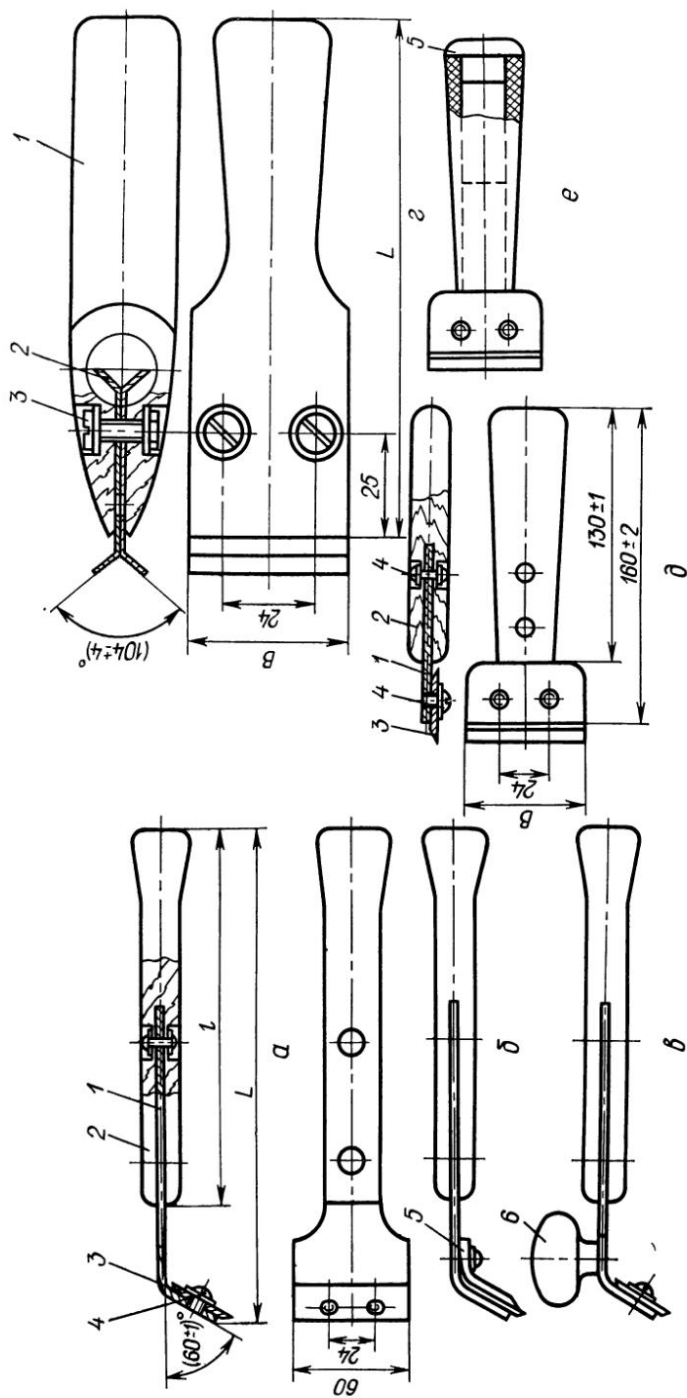
Рис. 59. Цикли:
