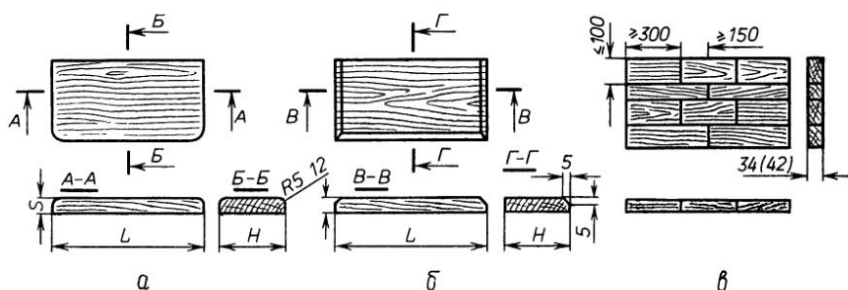
Рис. 27. Подоконные доски:
