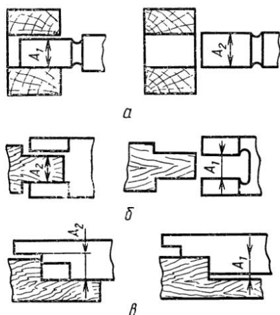
Рис. 64. Контроль размеров деталей при помощи предельных калибров: а — пробкой; б — скобой; в — уступоме-ром; A_1 — наименьший предельный раз-мер; A_2 — наибольший предельный размер
