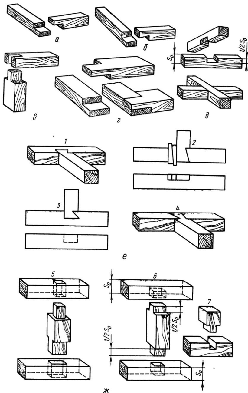
Рис. 18. Соединение брусьев:
