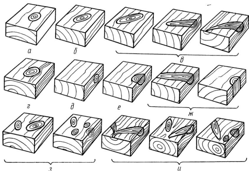
Рис. 3. Разновидности сучков:
