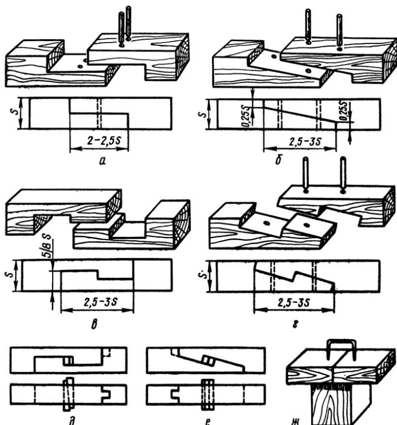
Рис. 17. Сращивание:
