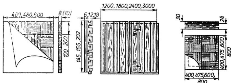
Рис. 9. Мозаичный паркет
