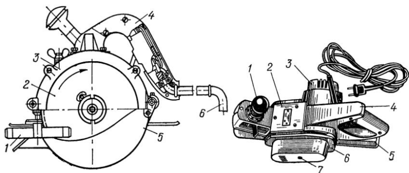
Рис. 40. Дисковая электропила ИЭ-5104:
