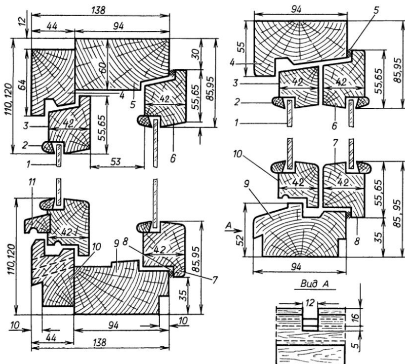
Рис. 23. Оконные блоки раздельной конструкции для жилых и общественных зданий (сечения по притворам):
