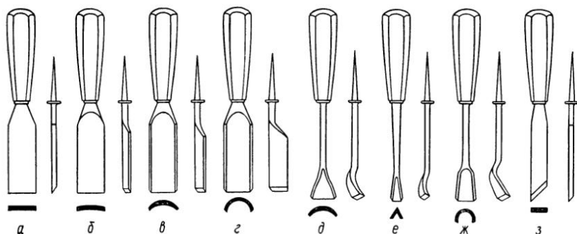
Рис. 62. Режущий инструмент для резьбы по дереву:
