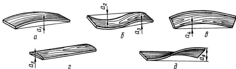
Рис. 6. Покоробленность:
