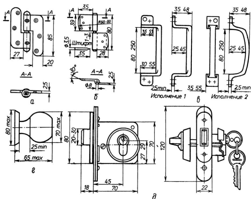
Рис. 21. Некоторые виды приборов для окон и дверей:
