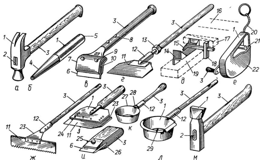
Рис. 60. Инструмент паркетчика:
