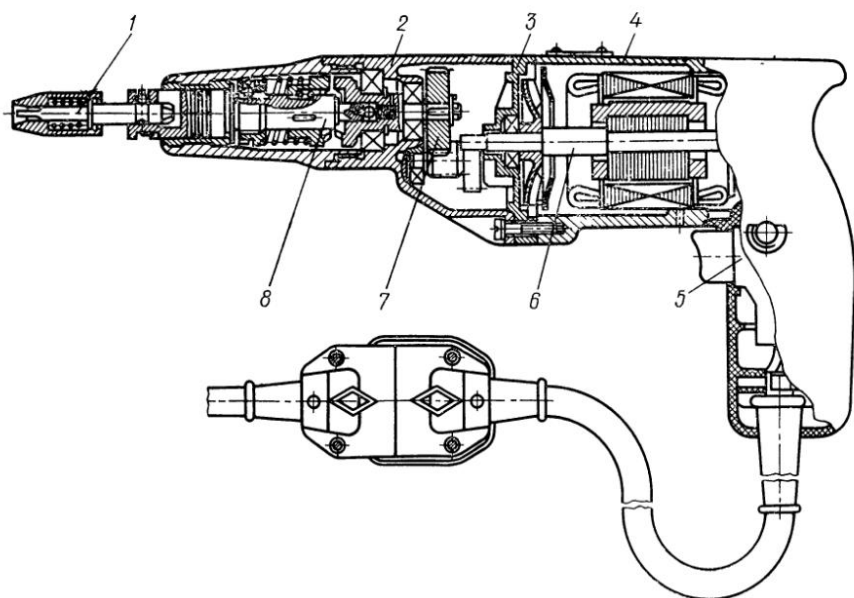
Рис. 44. Электрошурповерт ИЭ-3601Б:
