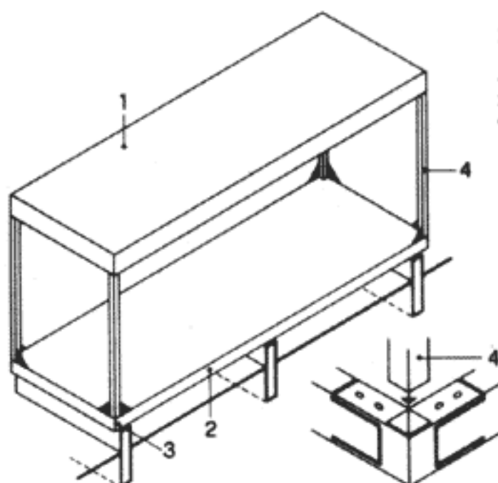
120 Зашцеplенная стальная стойка, шарнирно соединенная с деревянным щитом
