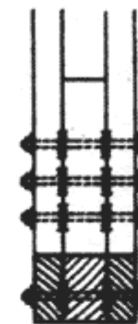
2 Двойная врубка зубом, усиленная накладками. Пример: опорный узел треугольной стропильной фермы с верхним поясом из двух и нижним из одного элемента
