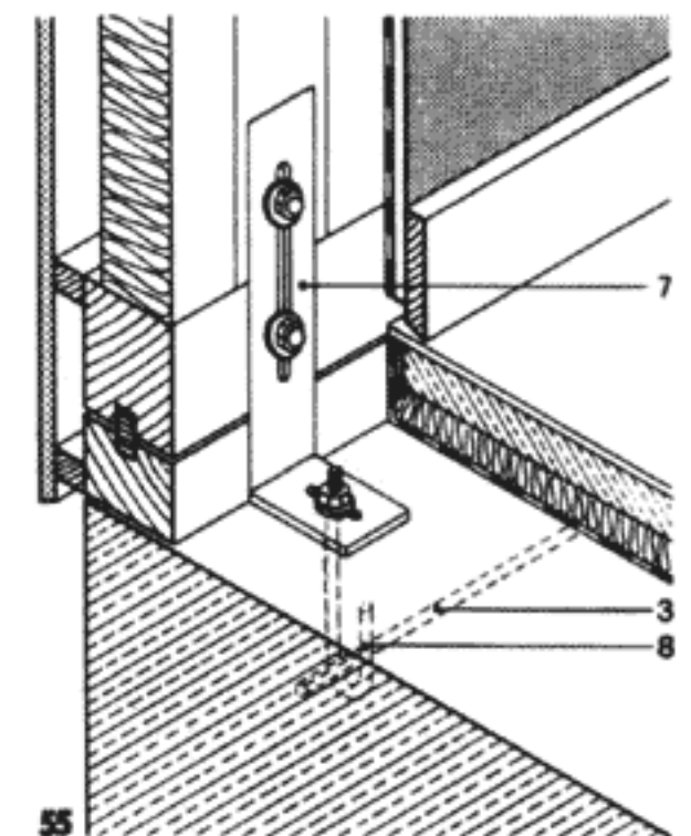
7 стальной уголок с продольными прорезями, легко юстируемый в двух направлениях 8 анкер в виде крюка 9 стойка 10 теплоизоляция
