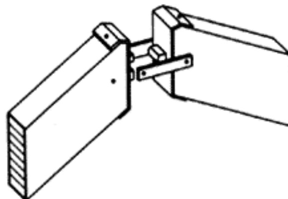
Торцовая накладка с выступами и боковыми страховыми накладками
