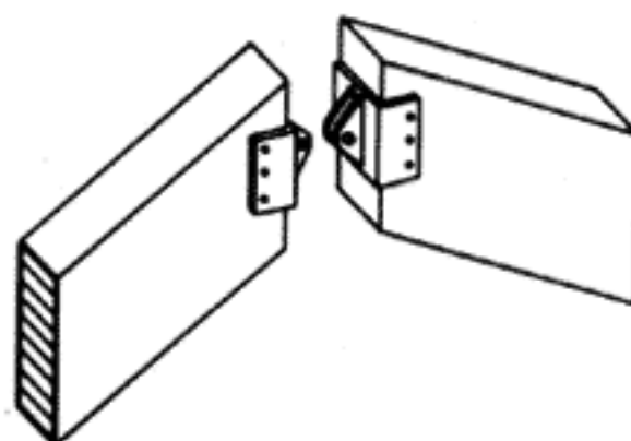
Стальной башмак с шарнирными болтами
