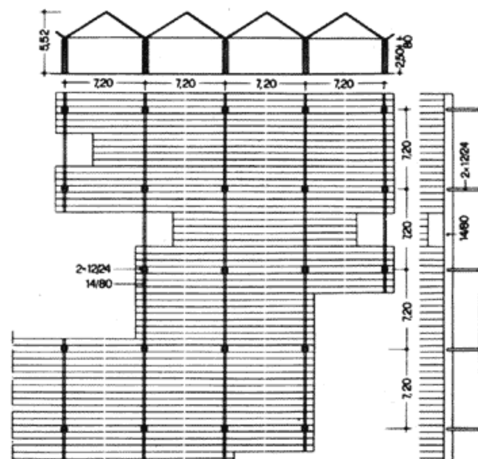
Несущая система
