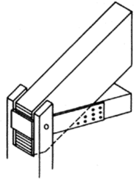
Крепление затяжек на опоре
