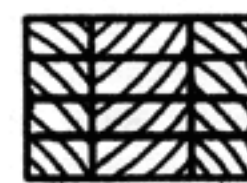
16а Односрезный гвоздевой шов
