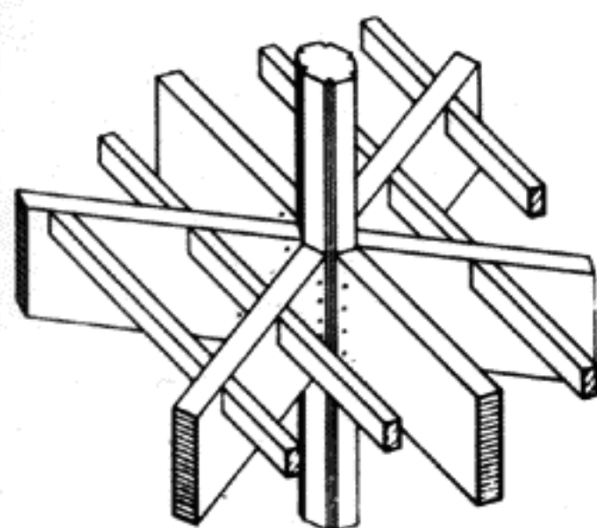
5 главные балки опираются на состыкованную стойку под углом 60^\circ
