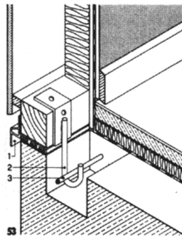
1 башмак из пластмассы 2 анкер нижней обвязки, приваренный к уголку 3 арматурная сталь
