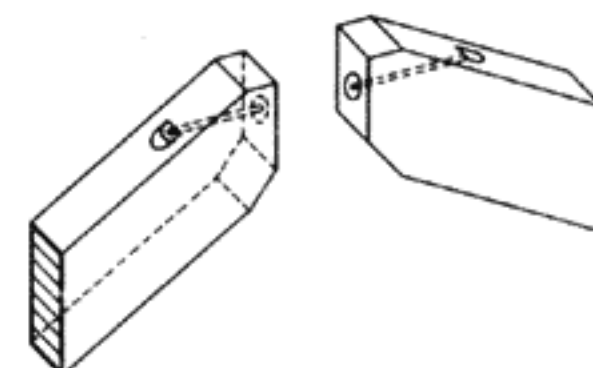
Сжатая пластинка из эластомера с торцевой шпонкой и сквозным болтом
