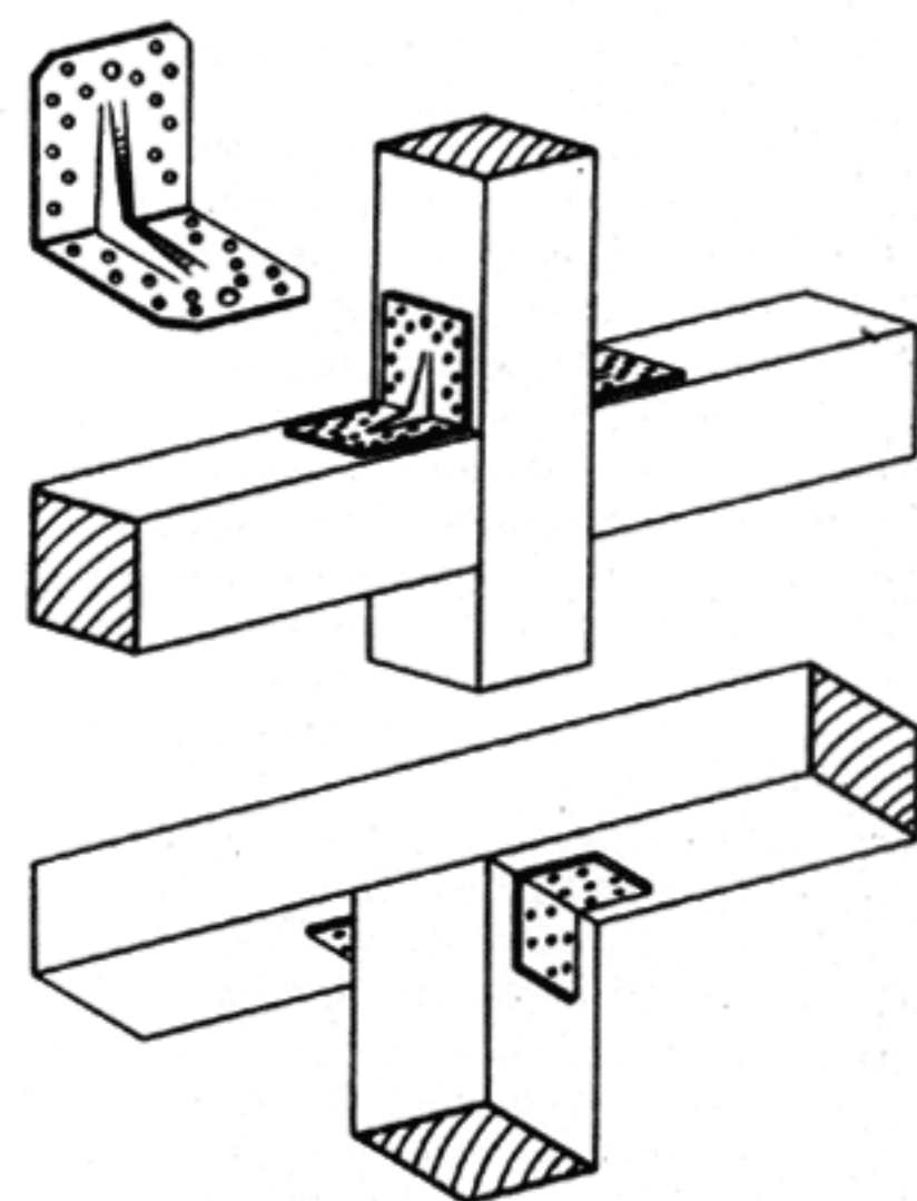
22 Угловая накладка
