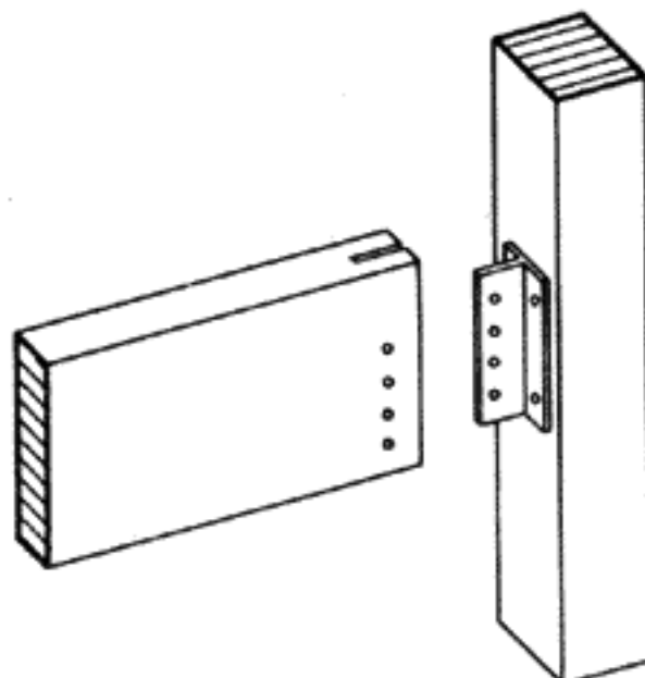
Балка уложена в башмак, прибитый гвоздями или глухарями к стойке
