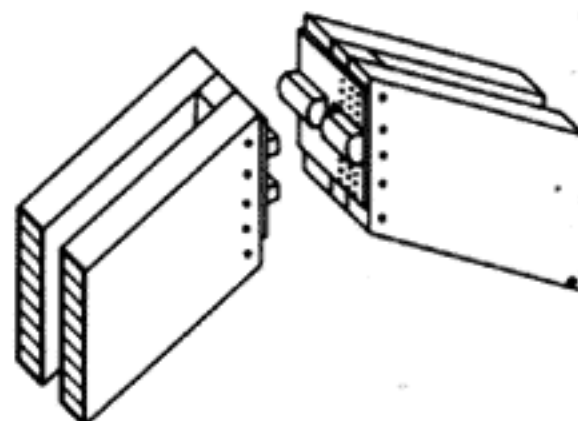
Торцовая накладка с выступами на спаренной балке. Фиксирование болтами через деревянную прокладку. Крепление деревянной прокладки нагелями
