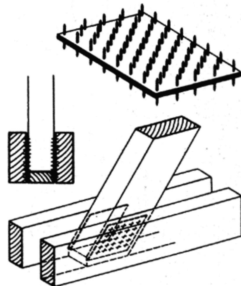
21б Соединение брусков с помощью плит «Мениг»
