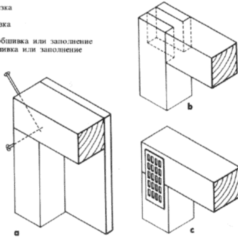
20 Соединение частей деревянной рамы с помощью: а — наклеенных древесностружечных плит при примыкании встык; б — шипов; с — оцинкованных гвоздевых плит при примыкании встык
