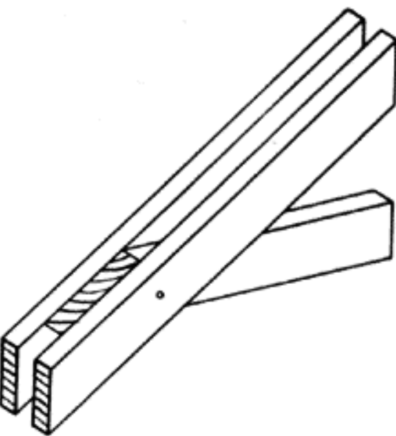
Одинарная затяжка парной стропильной, прикрепленная нагелями и болтами
