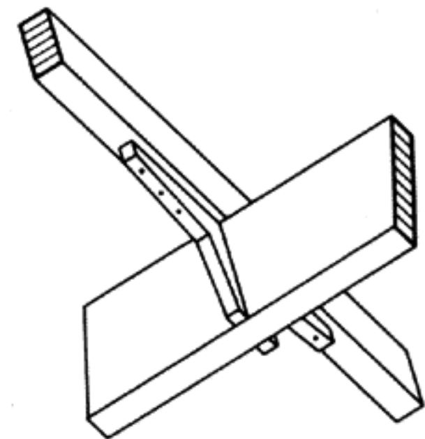
Уголковое крепление
