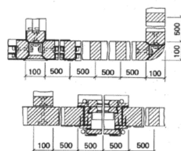
1 Дома в Финове: а — монтаж сборных стен; б — угол дома закрыт медной полоской; с — вертикальный разрез стенового элемента; д — горизонтальный разрез и соединение стеновых элементов
