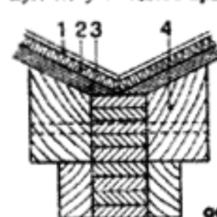
аа разрез через стропильную ногу в ендове крыши
