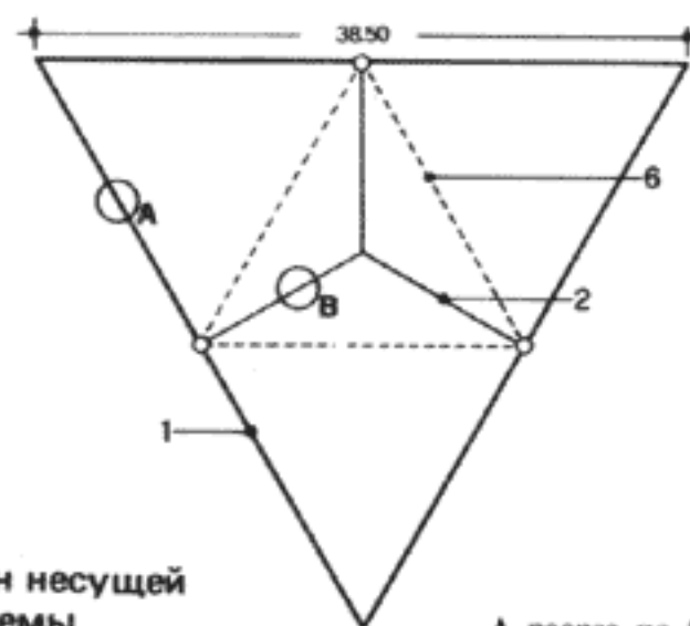
А разрез по бортовому элементу В разрез через ребро
