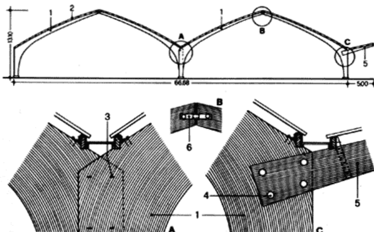
Гнутый угол из пакета клееных досок. Наугольник без несущей функции
