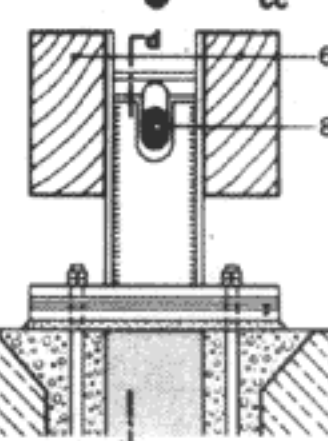
bb и cc узлы ферм dd и ee опорный узел
