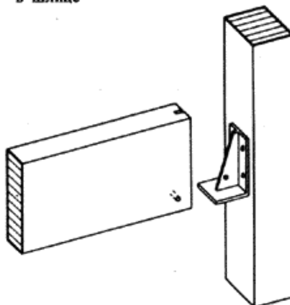
Балка опирается на уголок, усиленный кронштейном
