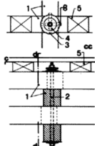
aa опора-бетонная обвязка cc и dd детали решетки из реек
