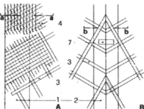
А разрез по бортовому элементу В разрез через ребро
