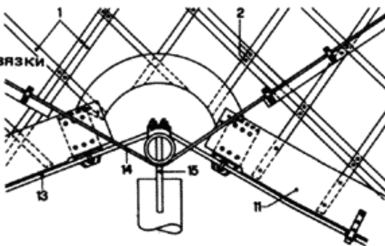
Опоры бортных канатов
