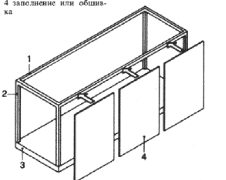
123 Пространственная рама над щитом пола с двухсторонней обшивкой и кровельным щитом
