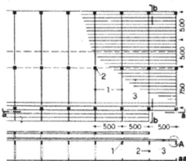
План расположения балок
