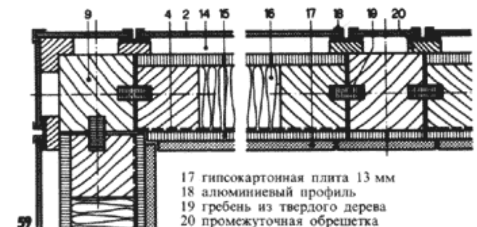
9 угловая стойка 10 деревянный гребень 11 деревянная рама 12 вентилируемое пространство 13 фанера 14 вентилируемое пространство 20 мм
