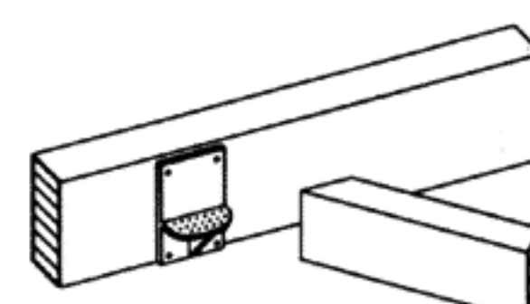
Приваренная к стальной пластинке полосовая сталь, заведенная в шлиц балки
