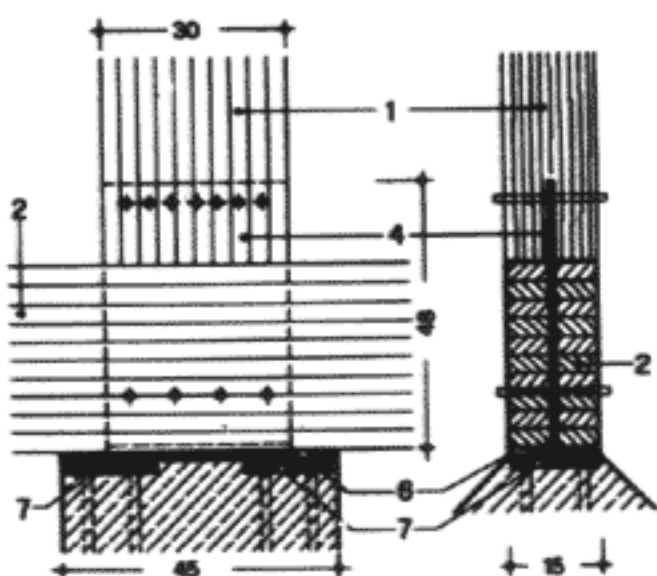
aa-cc крепление: поперечная балка-стойка-продольная балка внутри
