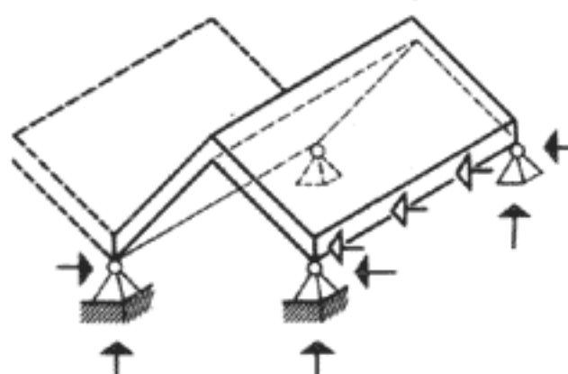
Реакции опор
