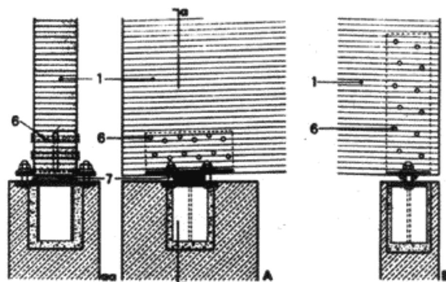
А подвижная опора В неподвижная опора
