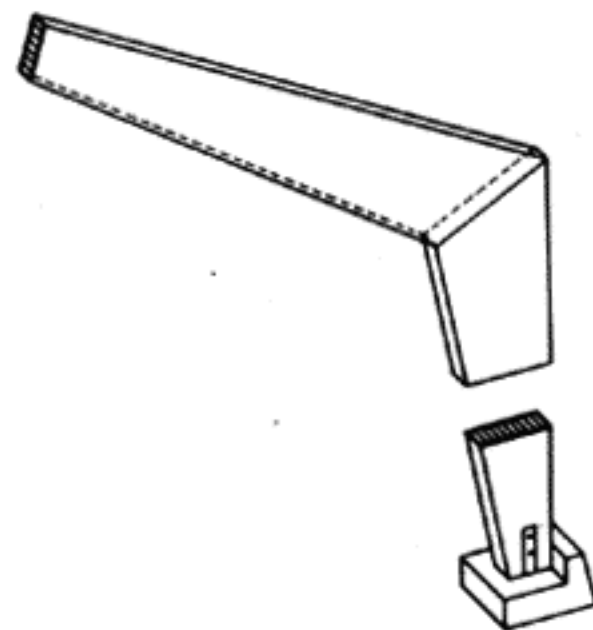
Угол рамы с зубчатым соединением
