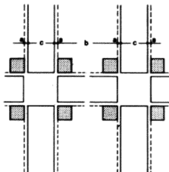
Скользящий шов
