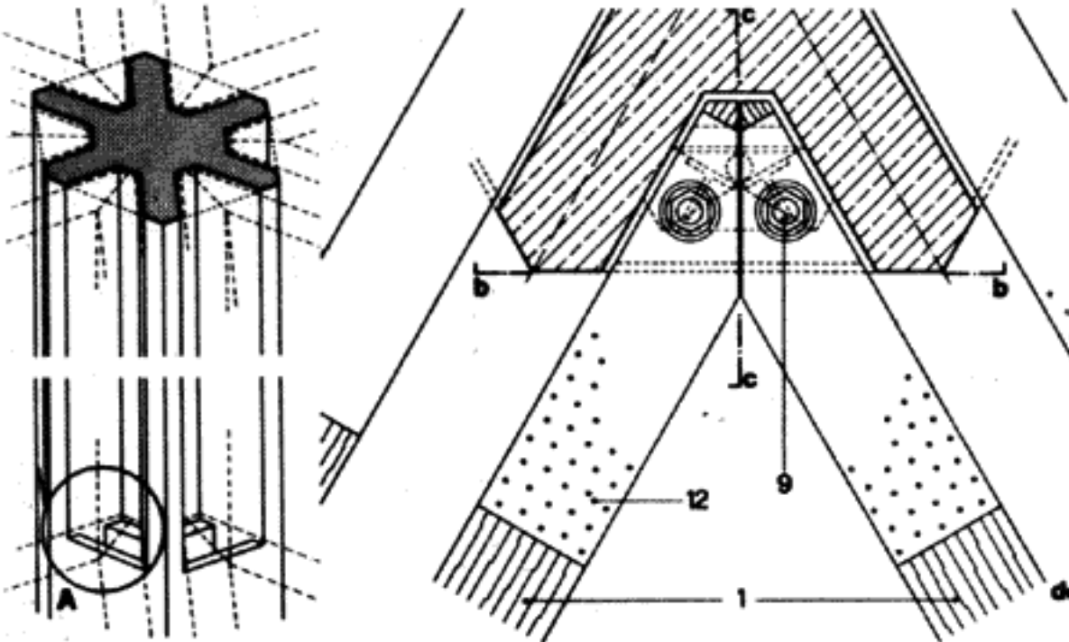
Присоединение балки к стойке
