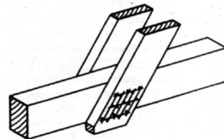
16c Четырехсрезный гвоздевой шов со стальными полосками
