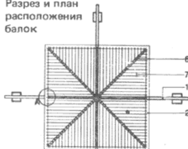
А опирание пирамидальной крыши на главную балку
