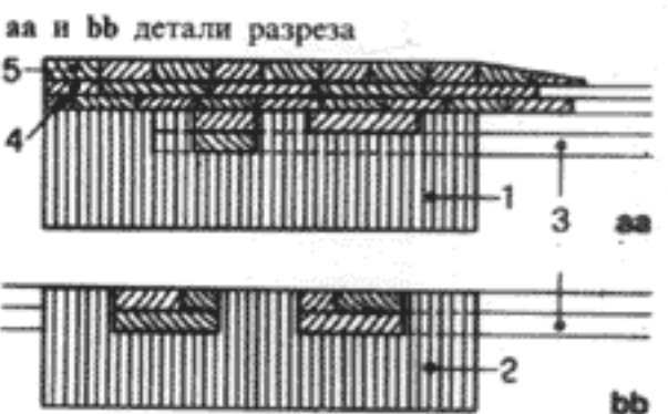
А разрез по бортовому элементу В разрез через ребро
