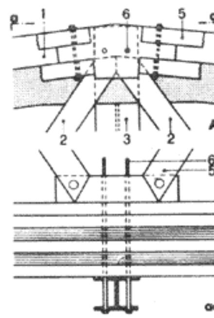
А коньковый узел с присоединением ветровых связей Б присоединение ветровых связей (аксонометрия)
