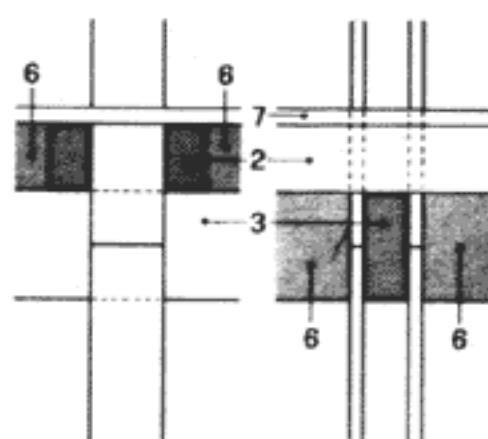
Балка на стойке двухэтажная
