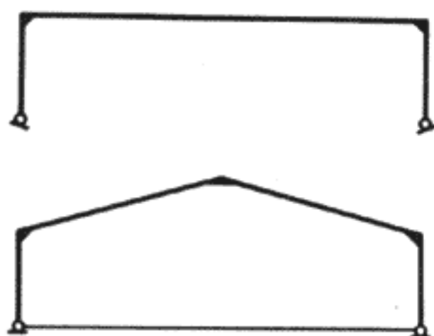
Реакции опор, соответствующие системе шарниров
