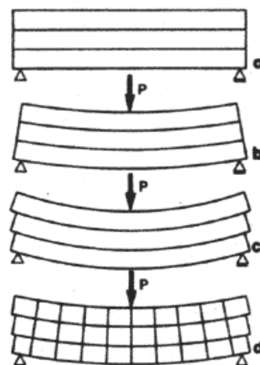
48 Составные изогнутые балки: а—ненагруженная балка (представлена выше обычной); б—балка с неподатливыми соединениями (в деревянных конструкциях—только пакет клееных досок); никаких сдвигов в контактных швах, максимальная прочность при изгибе; в—свободные, лежащие друг на друге отдельные брусья; максимальный сдвиг концевых сечений, минимальная прочность при изгибе; г—балки с податливыми соединениями; меньший сдвиг концевых сечений, прочность при изгибе между б и в
