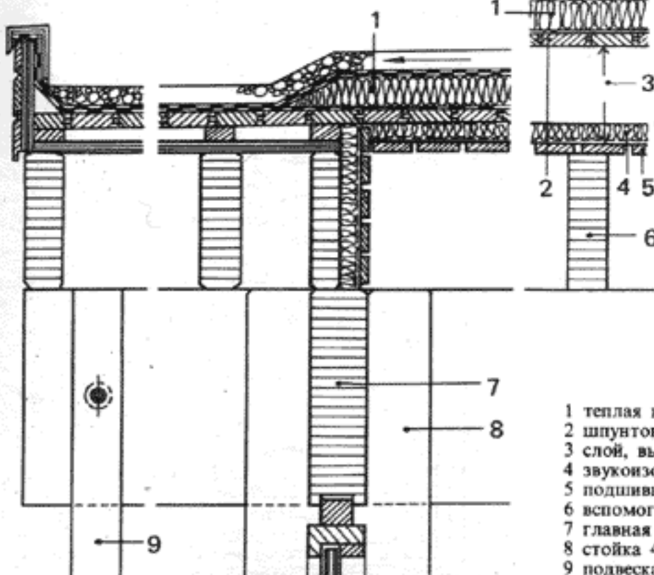
Деталь примыкания крыши
