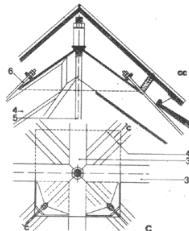
В узел пересечения главных балок с вершиной кровельной пирамиды
