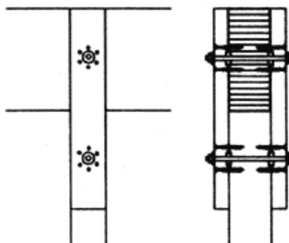
73 Шпонка особого вида с болтами и шестью дополнительными шурупами
