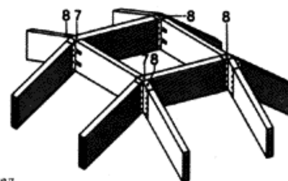
Приваренная к стальной пластинке полосовая сталь, заведенная в шлиц балки
