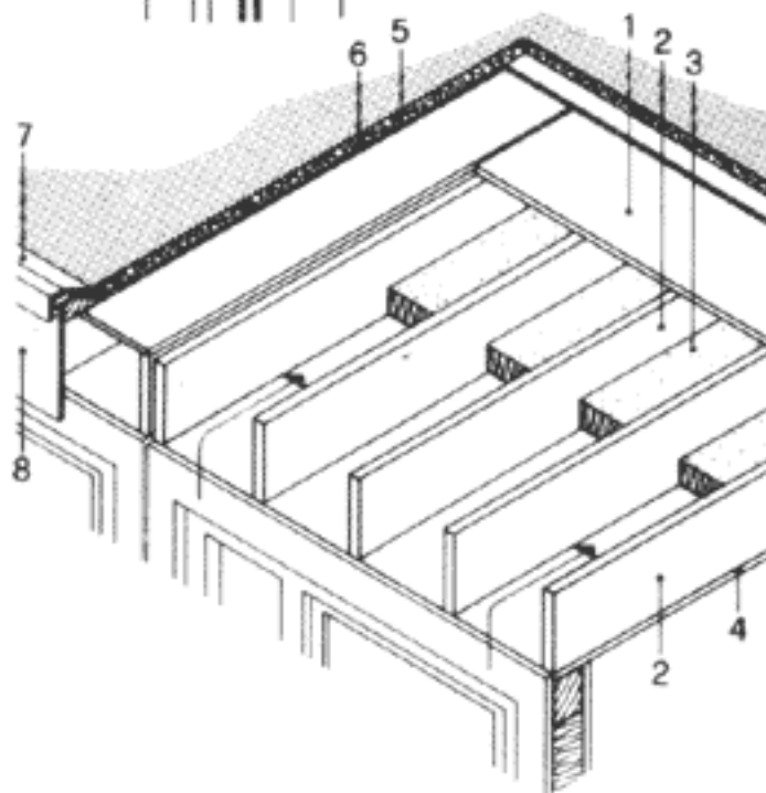
43 Кровельные щиты с несколькими средними ребрами b \approx 1,25 м
