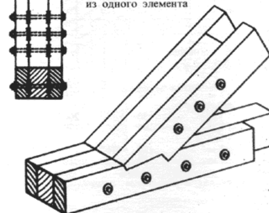
2 Двойная врубка зубом, усиленная накладками. Пример: опорный узел треугольной стропильной фермы с верхним поясом из двух и нижним из одного элемента
