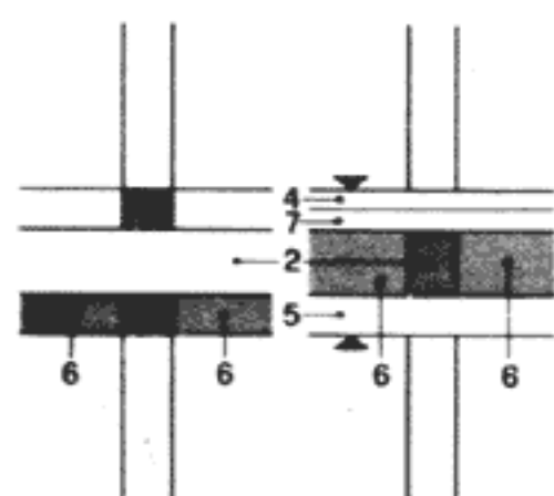
Фахверк
