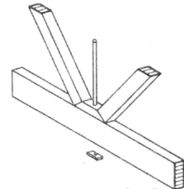
Сжатые диагонали с вружкой. Растянутые стойки с металлической шайбой
