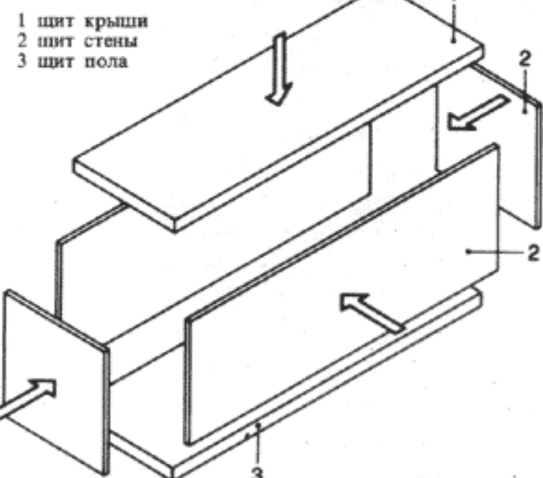
124 Изготовление щитов стен, кровли и пола на разных технологических линиях, затем соединение отдельных деталей в пространственную раму на главной линии
