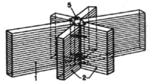
Аксонометрия узла
