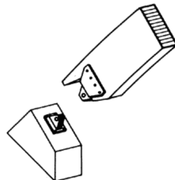
Стальной башмак с шарнирным болтом
