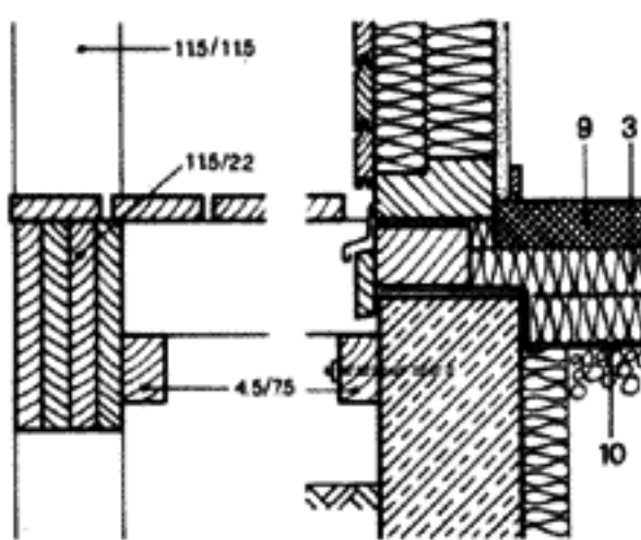
Горизонтальный разрез наружной стены с внешней и внутренней обшивкой
