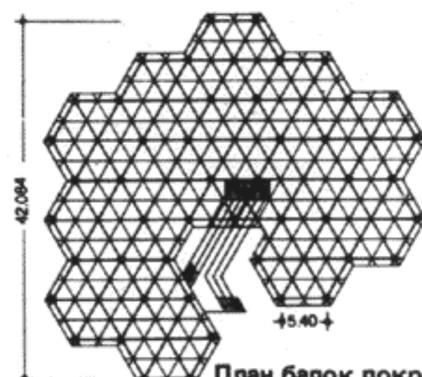
План балок покрытия
