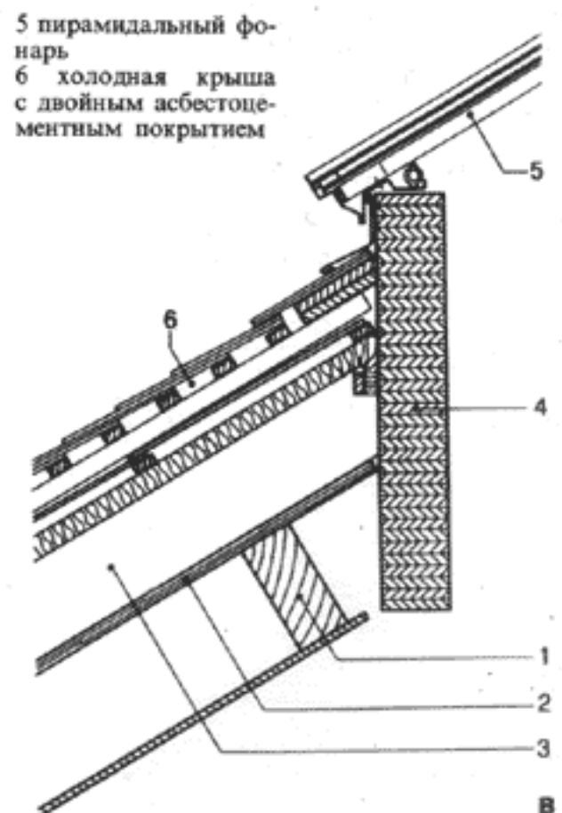
А карнизный узел В коньковый узел с пирамидальным фонарем
