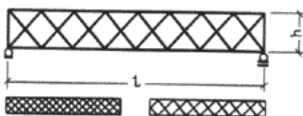
Ферма с параллельными поясами и ромбической решеткой: a = 2,5-6 м, l = 20-50 м, h = l/10-l/14 .
