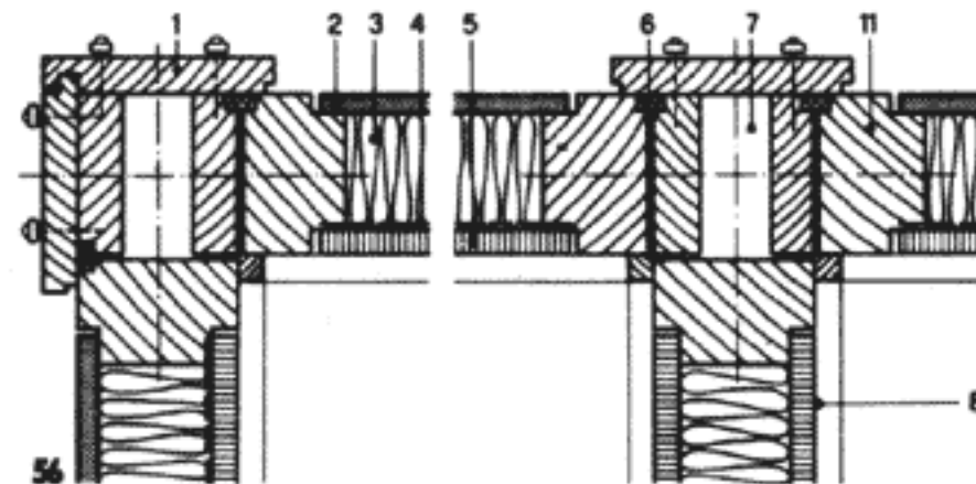
1 закрывающая доска 2 асбестоцементная плита 3 теплоизоляция 4 пароизоляция
