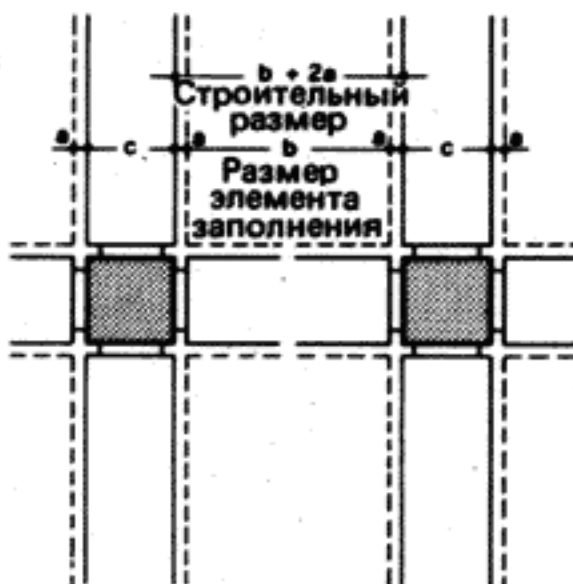
Шов встык
