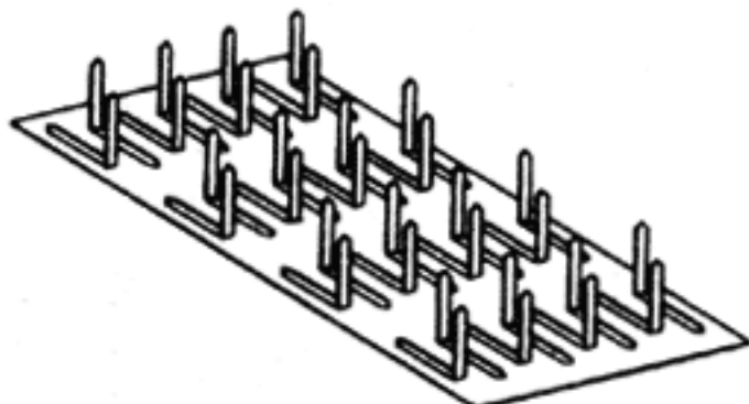
19б Гвоздевая плита системы «Ганг-нейл». Направление продольных щелей указывает на главное направление усилий в плите
