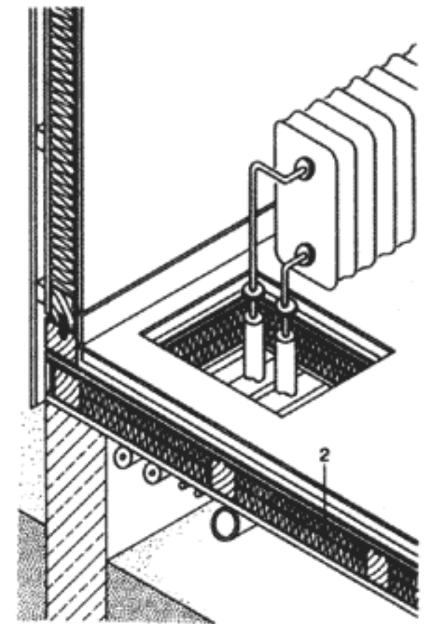
91 1 гидроизоляция 2 сборные щиты пола 3 усиленная теплоизоляция
