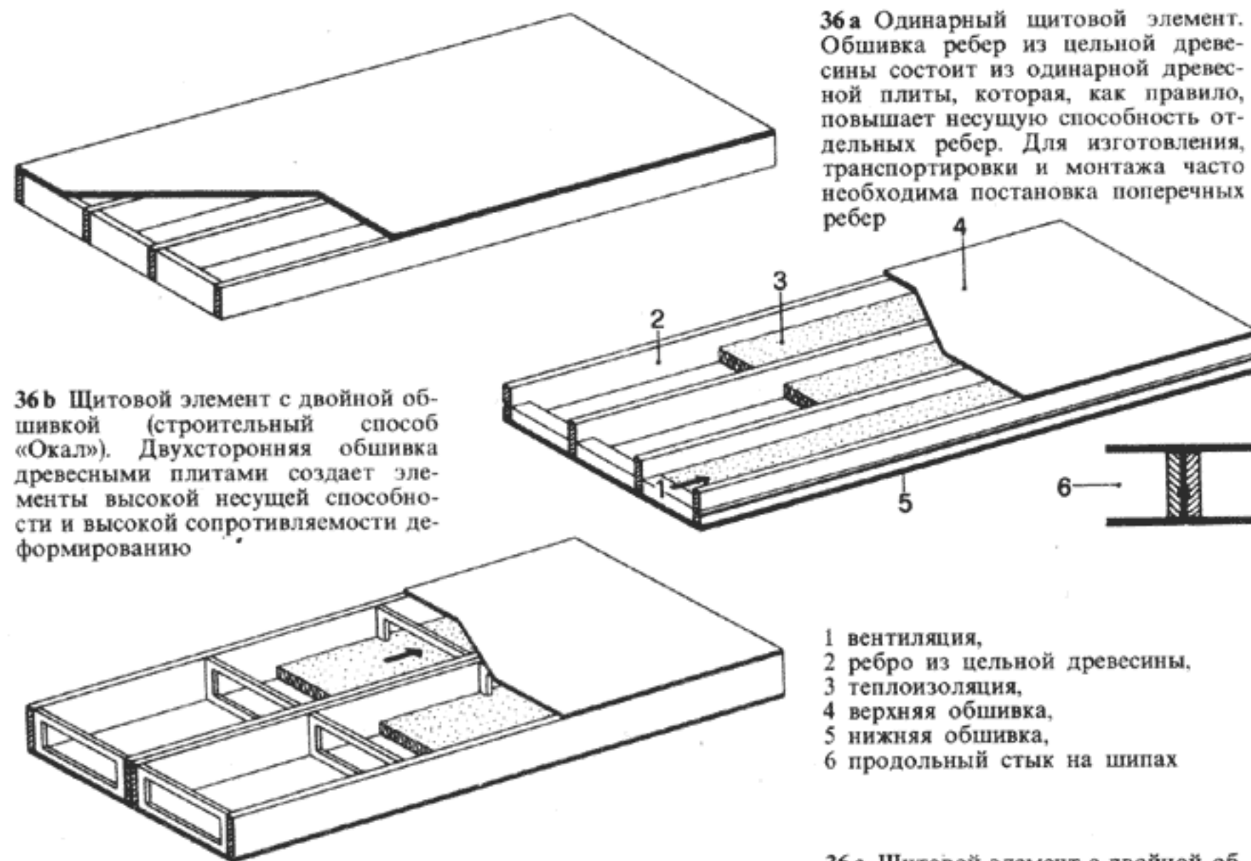
36с Щитовой элемент с двойной обшивкой (способ «Уайдфлекс»)
