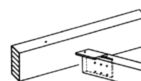
Опирается на деревянный черепной брусок, прикрепленный нагелями. Для страховки уложена сверху накладка из полосовой стали
