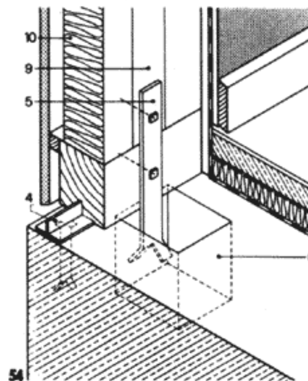
4 направляющий тавр 5 анкер из полосовой стали 6 прижимок
