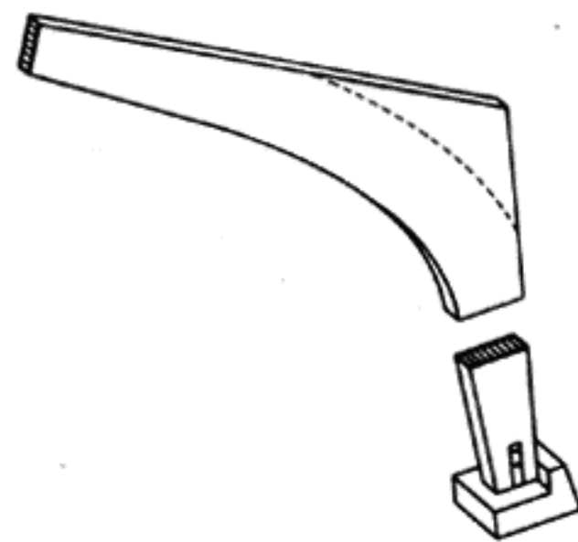
Гнутый угол из пакета клееных досок. Наугольник без несущей функции
