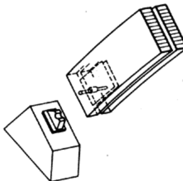
Двухветвевая арка с гвоздевыми планками внутри и шарнирной опорой
