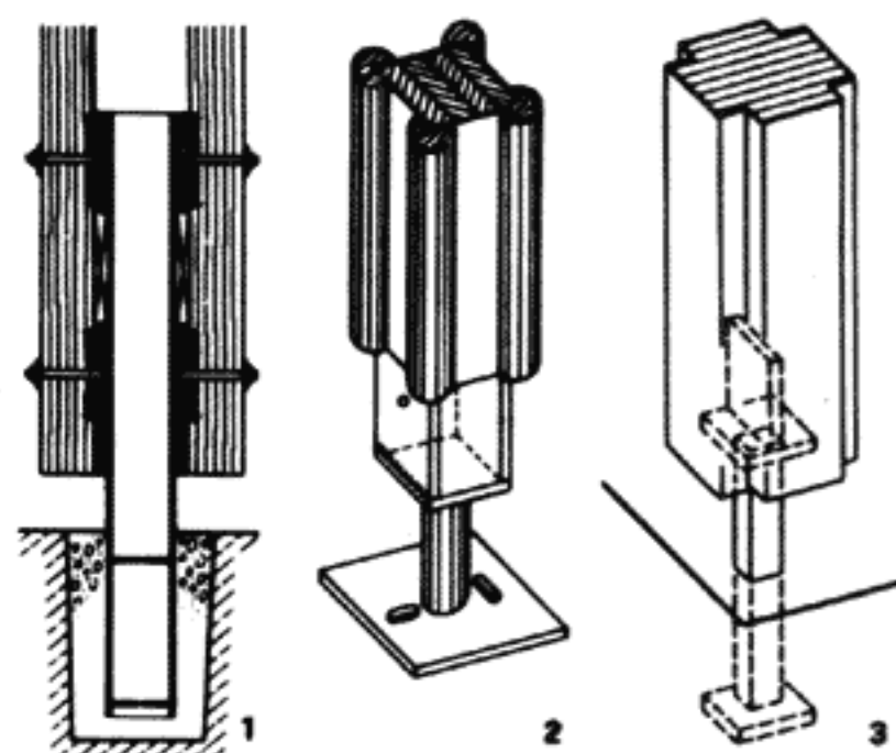
1 заземление составной стойки 2 опорная плита с овальными отверстиями для юстировки 3 стальная опора без юстировки
