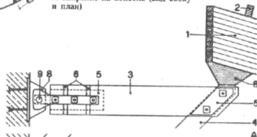
А опирание на консоль (вид сбоку и план)
