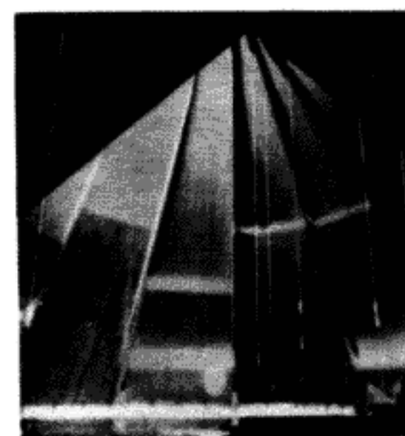
Опирается на деревянный черепной брусок, прикрепленный нагелями. Для страховки уложена сверху накладка из полосовой стали
