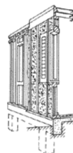
1 Дома в Финове: а — монтаж сборных стен; б — угол дома закрыт медной полоской; с — вертикальный разрез стенового элемента; д — горизонтальный разрез и соединение стеновых элементов
