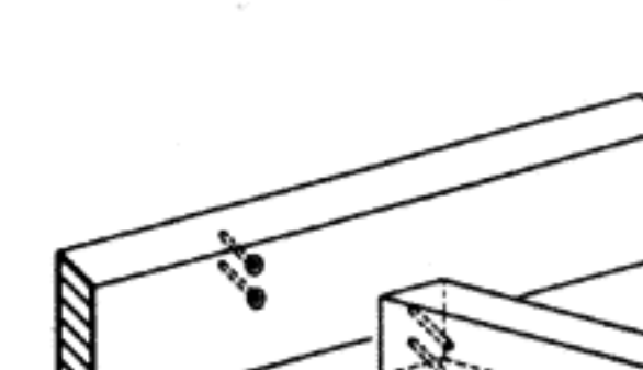
Шарнирное крепление с прикрепленной нагелями стальной прокладкой
