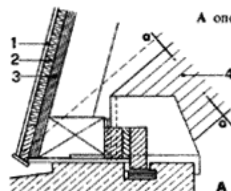
аа разрез через стропильную ногу в ендове крыши
