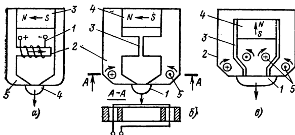
Рис. 2-34. Удерживающие поляризованные электромагниты.
