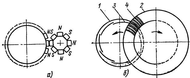
Рис. 2-21. Магнитные редукторы.
