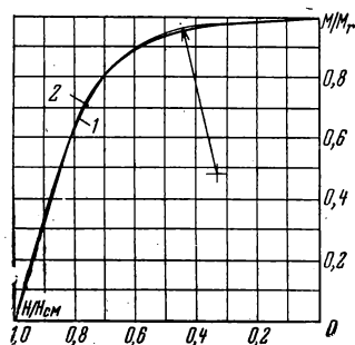
Рис. 1-59. Аппроксимация (1) кривой размагничивания сплава ПлЗ78 (2) дугой окружности и касательными.
