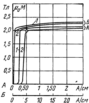
Рис. 9-8. Кривые индукции намагниченности ленты железкобальтовых сплавов толщиной 0,1 мм.
