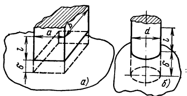
Рис. 3-49. К расчету проводимости между элементами. а — призмы; б — цилиндра и плоскости.
