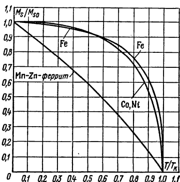
Рис. 1-5. Зависимость относительной намагниченности насыщения M_s/M_{s0} ферро- и ферримагнетиков от относительной температуры T/T_K .
