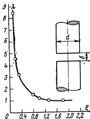
Рис. 3-48. К расчету проводимости между торцевыми поверхностями с учетом выпучивания магнитного поля.
