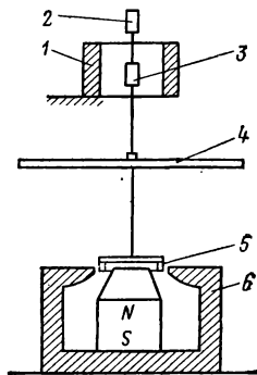
Рис. 2-30. Опора Штейнгривера.
