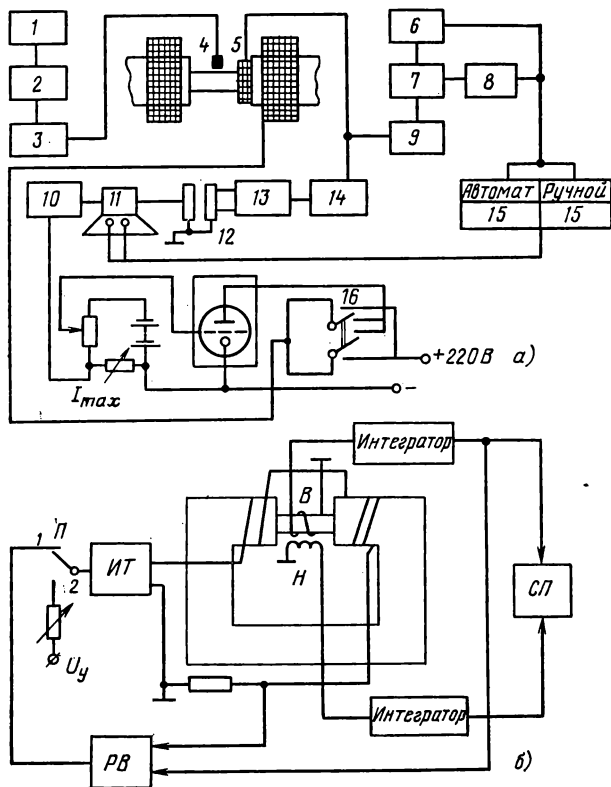
Рис. 10-7. Схемы установок.
