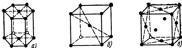
Рис. 1-7. Элементарные ячейки кристаллических решеток. а — гексагональная; б — объемно-центрированная; в — гранецентрированная.
