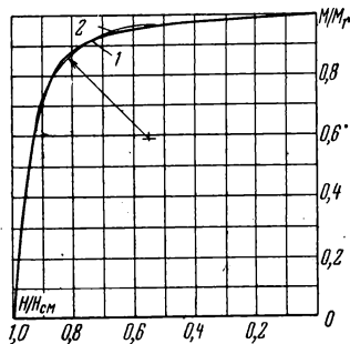
Рис. 1-60. Аппроксимация (1) кривой размагничивания литого сплава ЮНДК35Т5 (2) дугой окружности и касательными.
