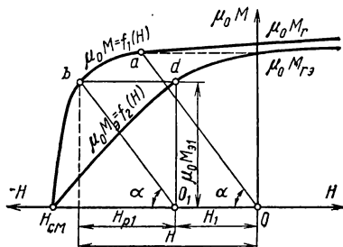
Рис. 3-6. Построение кривой намагничивания эллипсоида.
