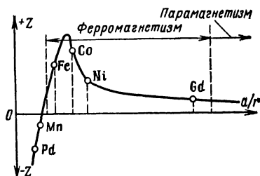
Рис. 1-2. Зависимость интеграла обменной энергии от отношения межатомного расстояния a к радиусу r незаполненной электронной подоболочки.
