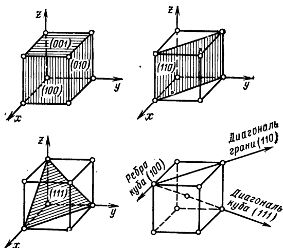
Рис. 1-8. Обозначение различных плоскостей и направлений в кубических кристаллах с помощью индексов Миллера.
