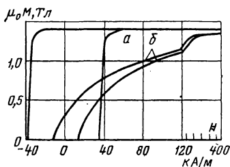
Рис. 1-10. Петли гистерезиса сплава аликнио.
