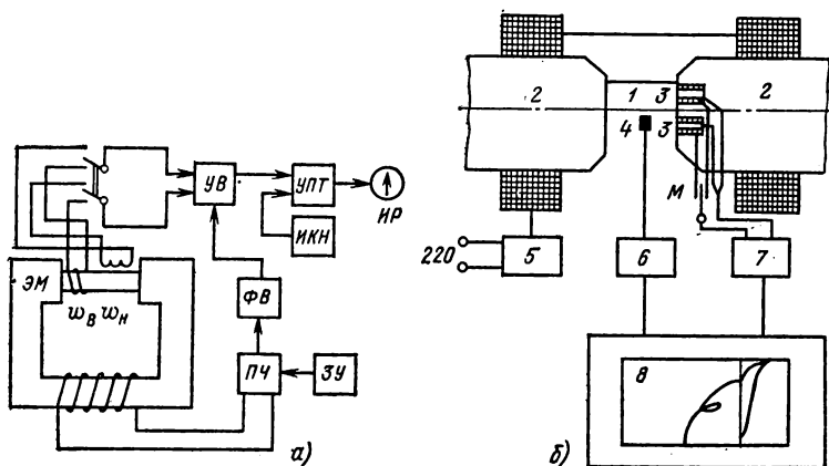
Рис. 10-6. Схема компенсационного устройства для испытания ПМ (а); схема установки Штейнгривера (б).
