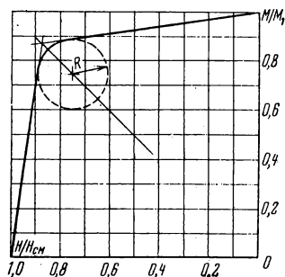
Рис. 1-61. Аппроксимация (1) кривой размагничивания феррита 19БА260 (2) дугой окружности и касательными.
