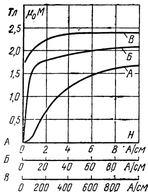
Рис. 9-6. Кривая индукции намагниченности сплава 27KH.
