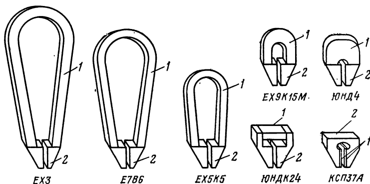
Рис. 1-65. Сравнительные размеры постоянных магнитов из различных материалов.
