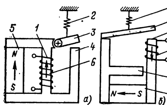
Рис. 2-33. Поляризованные электромагниты исполнительных механизмов.
