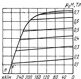
Рис. 6-11. Кривая размагничивания прутка диаметром 5 мм сплава ПлК78.
