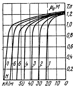
Рис. 6-8. Влияние упругого растяжения на кривые размагничивания проволоки из сплава 52К11Ф. Кривые измерены при нагрузках. 1 — без нагрузки; 2 — 510 МПа; 3 — 1010 МПа; 4 — 1520 МПа; 5 — 2030 МПа; 6 — 2540 МПа; 7 — 3050 МПа.
