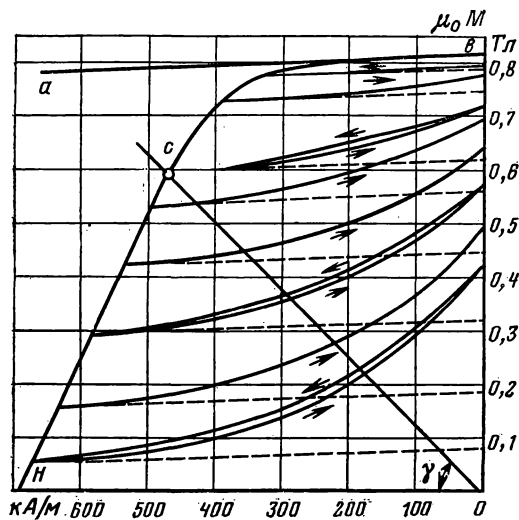
Рис. 1-64. Петли циклов магнитного возврата, снятые с образца РЗМ SmCo₅.
