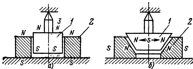
Рис. 2-23. Радиально-аксиальные подшипники.
