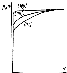
Рис. 1-9. Кривые намагничивания монокристалла железа в разных направлениях.
