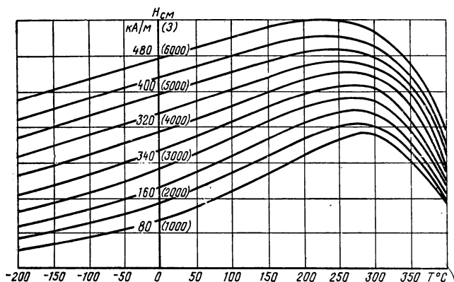
Рис. 7-3. Зависимость значения коэрцитивной силы H_{cm} от температуры.
