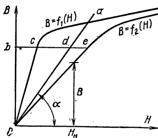
Рис. 3-29. Построение кривой намагничивания стенок экрана.
