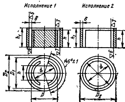
Рис. 2-38. Нормализованные магнитные системы с внутренним неподвижным магнитом,
