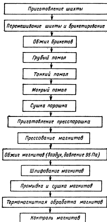
Рис. 7-2. Схема технологического процесса производства магнитов из ферритов кобальта.
