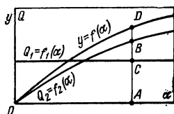
Рис. 3-31. Характеристика магнитной системы с разделенными полями.
