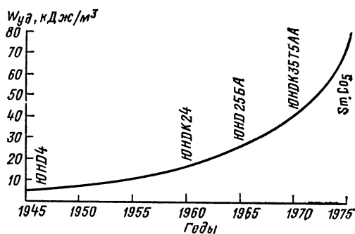
Рис. 1-66. Характеристика прогресса в области усовершенствования магнитно-твердых материалов.
