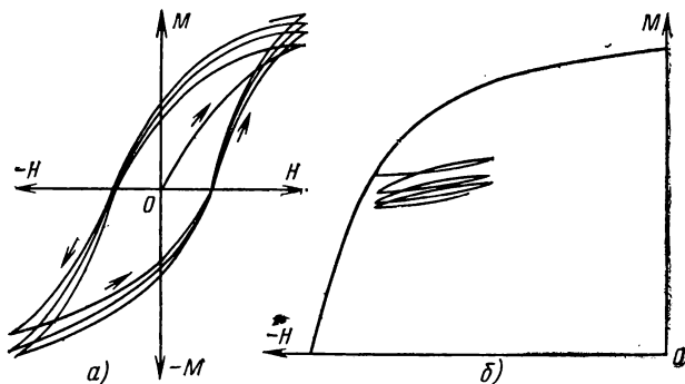
Рис. 1-17. Магнитная аккомодация.
