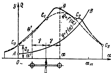
Рис. 3-34. Метод базисного участка. Общий случай.
