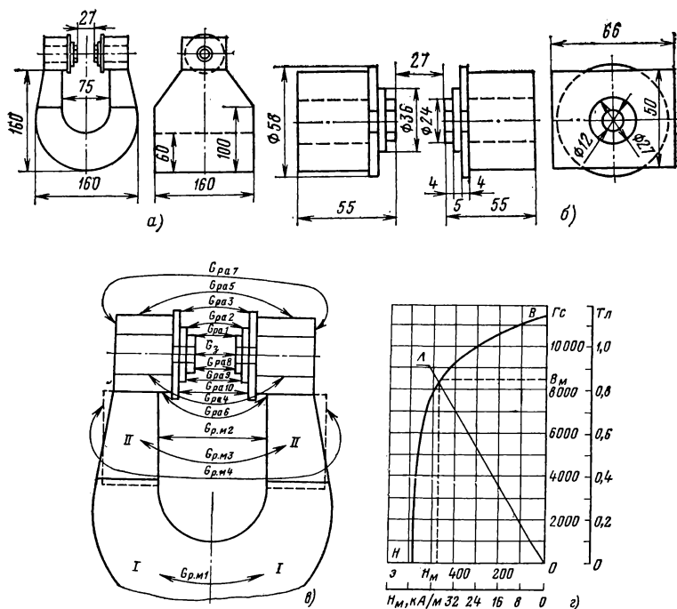
Рис. 3-40. К расчету П-образных односвязных магнитных систем. а — эскиз магнитной системы; б — эскиз полюсных наконечников; в — схема путей рассеяния магнитного потока в односвязной системе; г — кривая размагничивания сплава типа ЮНДК24.
