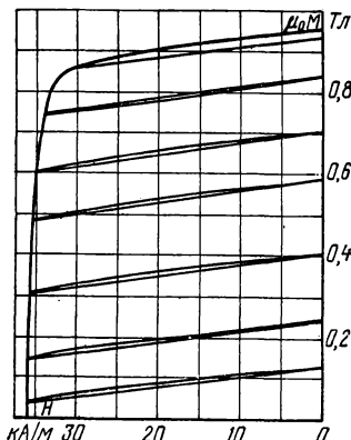
Рис. 6-8. Влияние упругого растяжения на кривые размагничивания проволоки из сплава 52К11Ф. Кривые измерены при нагрузках. 1 — без нагрузки; 2 — 510 МПа; 3 — 1010 МПа; 4 — 1520 МПа; 5 — 2030 МПа; 6 — 2540 МПа; 7 — 3050 МПа.
