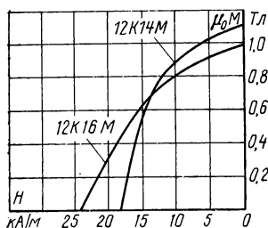
Рис. 6-13. Кривые намагничивания поковок из сплавов типа комол.
