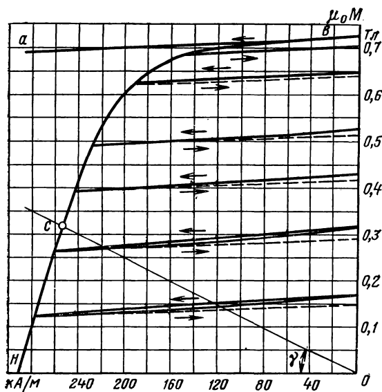
Рис. 1-63. Петли циклов магнитного возврата, снятые с образца сплава ПЛК78.
