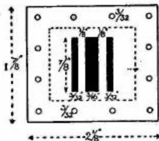
FIG. 59.—Valve plate.
