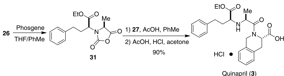
Scheme 10.8.
