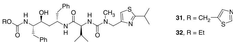
Scheme 2.9.
