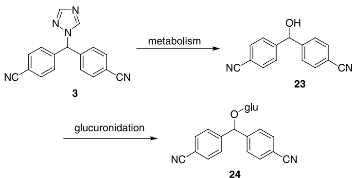
Scheme 3.4.
