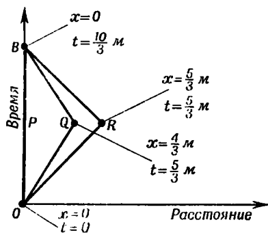
Р и с. 21. Сравнение трех разных мировых линий, связывающих события O и B . Резкие изменения скорости в событиях Q и R изображают предельный случай использования малых («противоударных») часов.
