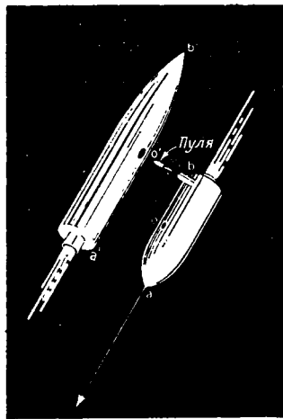
Р и с. 43. Наблюдатель в системе O' ожидает, что снаряд, выпущенный, когда точки a и a' совпадали, попадет в другой корабль.
