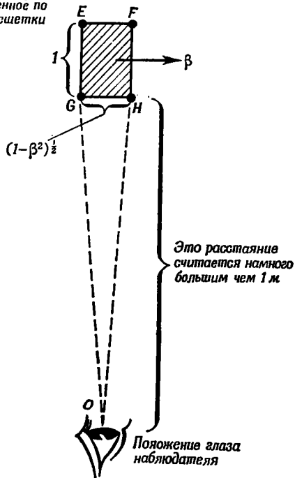
Р и с. 72. Положение глаза наблюдателя, визуально исследующего пролетающий мимо него «куб».
