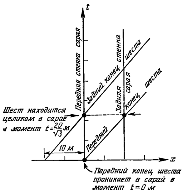
Р и с. 144. Пространственно-временная диаграмма в системе отсчета сарая.
