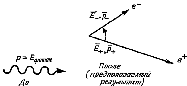
Р и с. 156. Диаграмма предполагаемой реакции: слева одиночный фотон до реакции, справа — предполагаемый результат реакции (пара электрон и позитрон). Реакция не идет.
