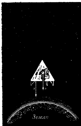
Р и с. 4. Космический корабль, свободно падающий вблизи Земли.
