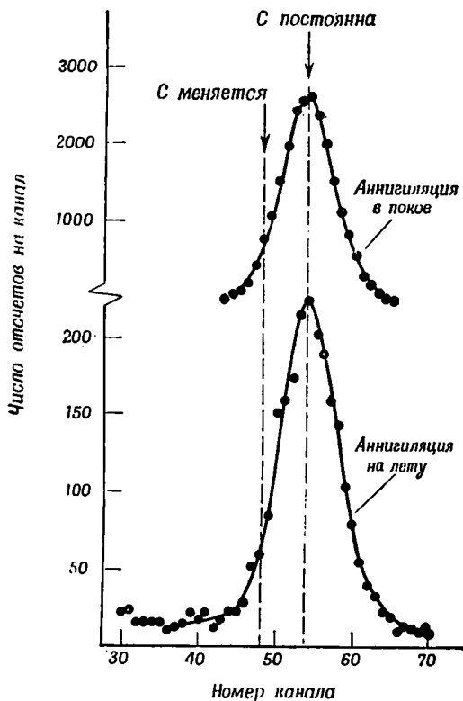
Р и с. 123. Результаты эксперимента по проверке постоянства скорости света, выполненного Д. Саде.
