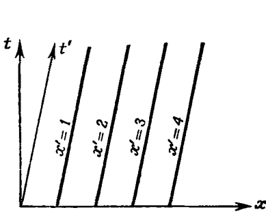
Р и с. 64. Положение на диаграмме пространства-времени в лабораторной системе отсчета оси времени системы отсчета ракеты.
