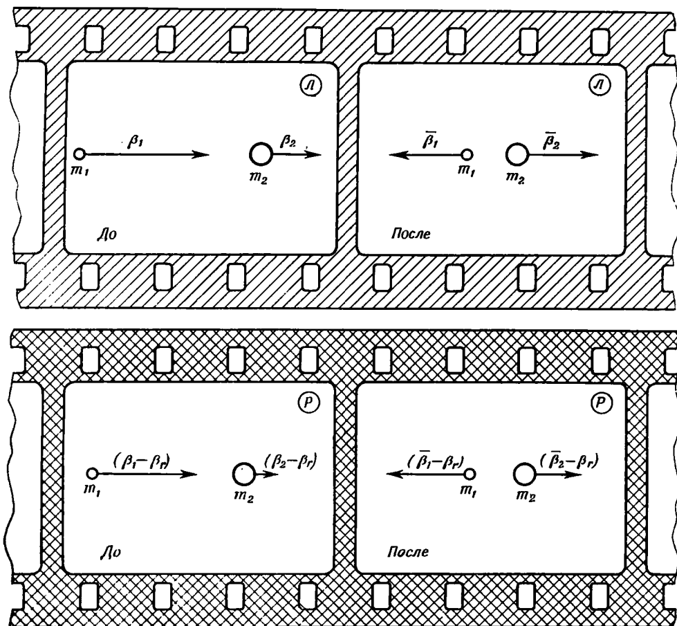
Р и с. 102. Анализ упругого лобового столкновения частиц разных масс в ньютоновской механике. Скорости частиц до и после соударения в лабораторной системе отсчета (верхний рисунок) и в системе отсчета ракеты (нижний рисунок), найденные по ньютоновскому закону сложения скоростей.
