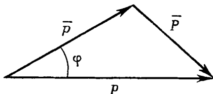
Р и с. 109. Диаграмма сохранения импульса при комптоновском рассеянии. Вспомните закон косинусов:
