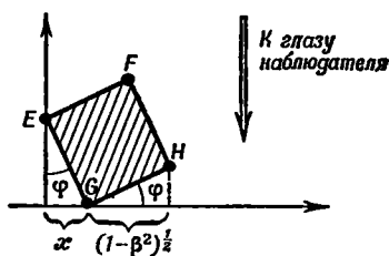
Р и с. 74. Как этот наблюдатель может истолковать свои визуальные наблюдения (проекцию рис. 73).
