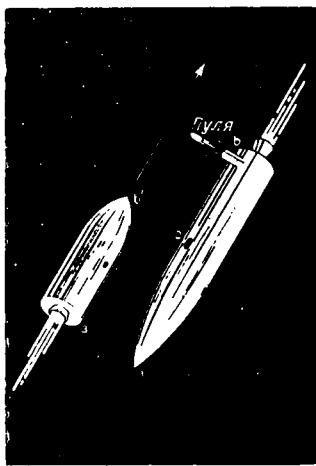
Р и с. 42. Наблюдатель в системе O ожидает, что снаряд, выпущенный, когда точки a и a' совпадали, не попадет в другой корабль.
