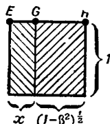
Р и с. 73. Что видит наблюдатель, смотря снизу вверх.
