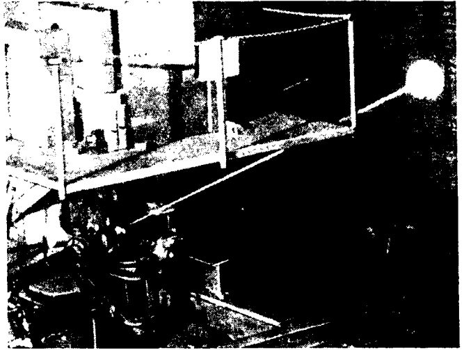
Р и с. 63. Черенковское излучение, генерируемое пучком электронов, движущихся в воздухе при энергии 700 Мэв.
