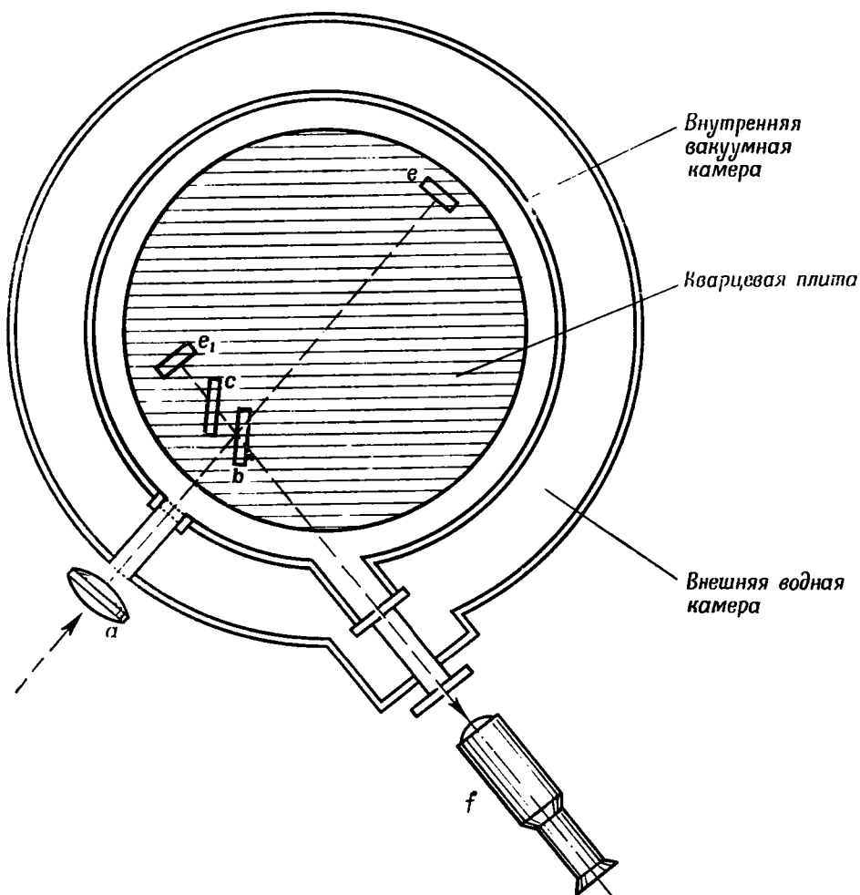
Р и с. 49. Схематическое изображение установки, использованной в эксперименте Кеннеди — Торндайка.
