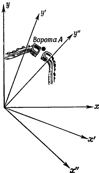
Р и с. 16. Относительное расположение координатных осей, соответствующее выбору направления на север дневного, ночного и некоего третьего землемеров.
