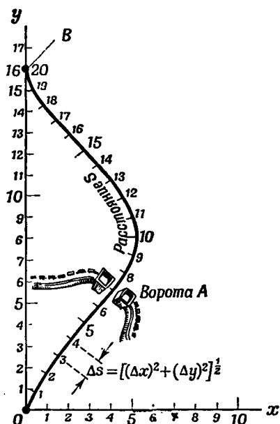
Р и с. 19а. Расстояние вдоль искривленного пути, начинающегося на городской площади. Заметим, что полное расстояние вдоль искривленного пути от точки O до точки B больше, чем расстояние по прямому пути (ось y ) от точки O до точки B .
