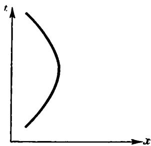
Р и с. 80. Мировая линия частицы, на которую действует сила.
