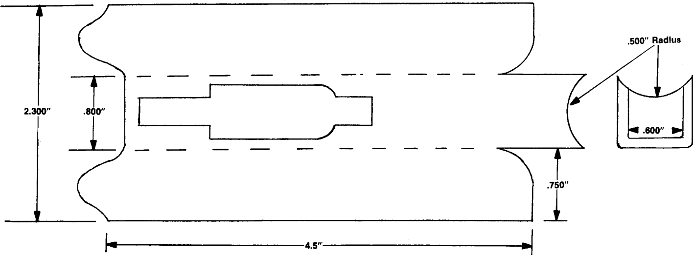
FRAME TEMPLATE
