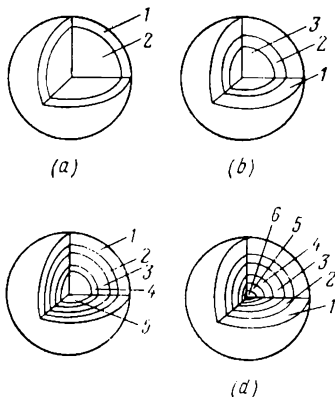
Fig. 9.4. Targets for laser fusion: (a) 1) glass shell, 2) gaseous D + T fuel; (b) 1) polytetrafluorethylene, 2) glass, 3) gaseous D + T fuel; (c) 1) beryllium, 2) tantalum shell, 3) foam plastic, 4) gold shell, 5) D + T fuel; (d) 1) LiH shell, 2) tantalum shell, 3) frozen layer of D + T fuel, 4) cavity, 5) gold, 6) D + T fuel.
